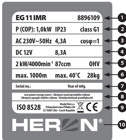
4. ábra. Gépcímke (1. ábra, 3-as tétel)
