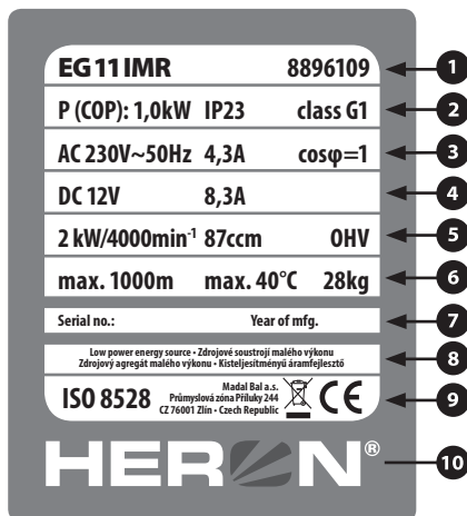
Obr. 4, Technický štítok (obr. 1 pozícia 3)
