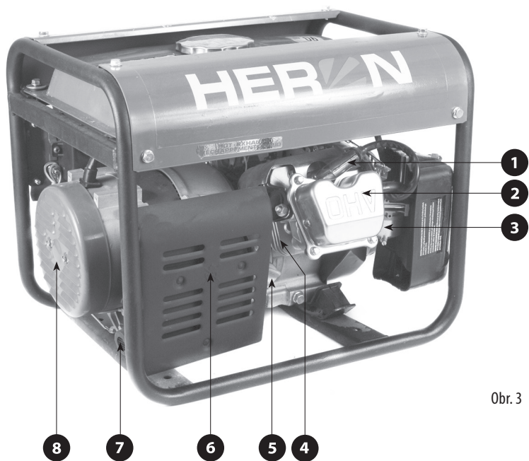
Obr.3, pozice-popis
