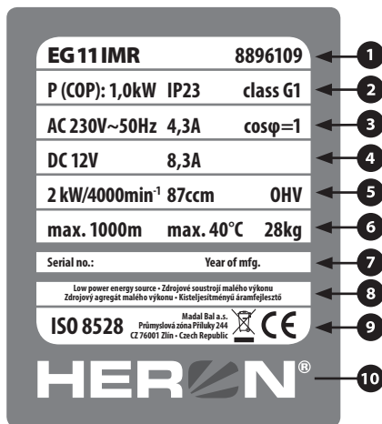
Obr. 4, Technický štítek (Obr.1, pozice 3)
